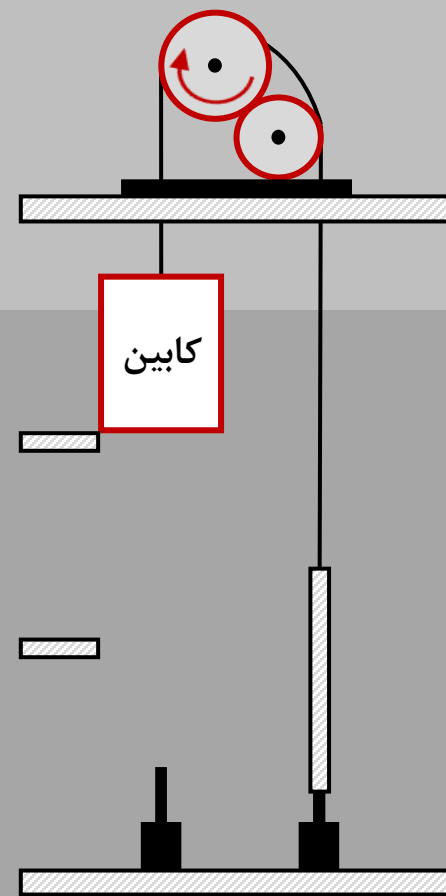
آسانسور کششی
