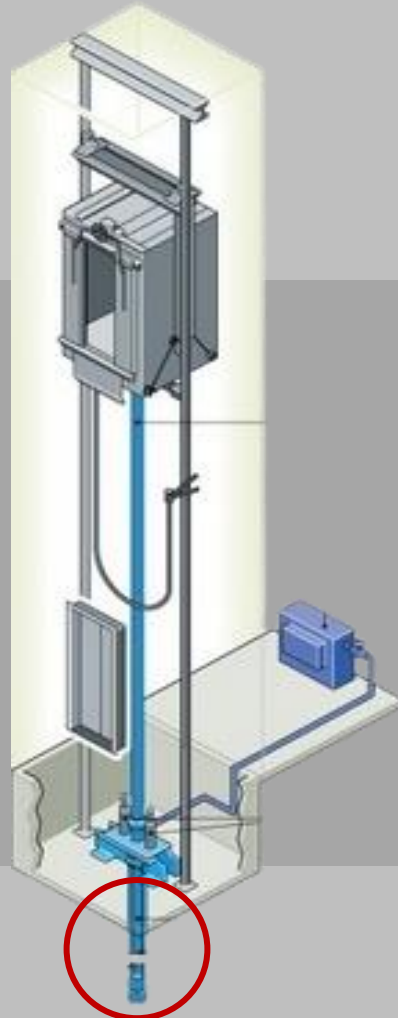
جک مستقیم از زیر
