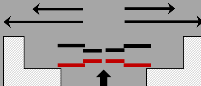
درب سنترال چهارلته وسط بازشو
